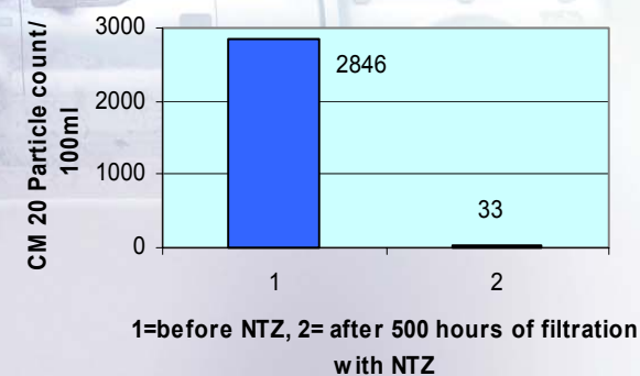
Particles > 15 micron
