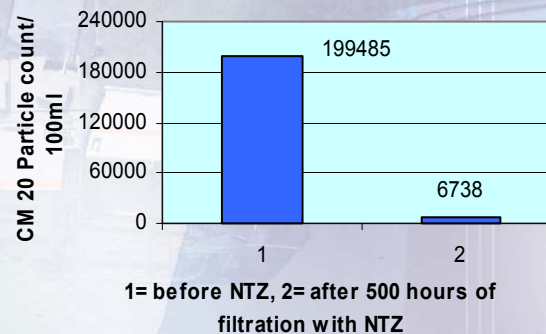
Particles > 5 micron
