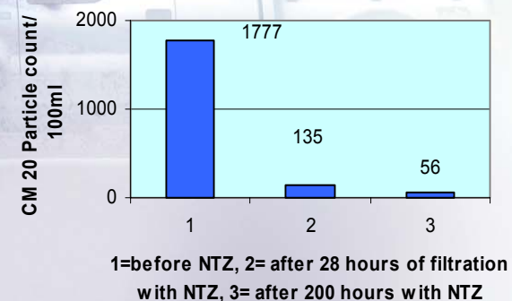
Particles > 15 micron
