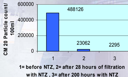
Particles > 5 micron
